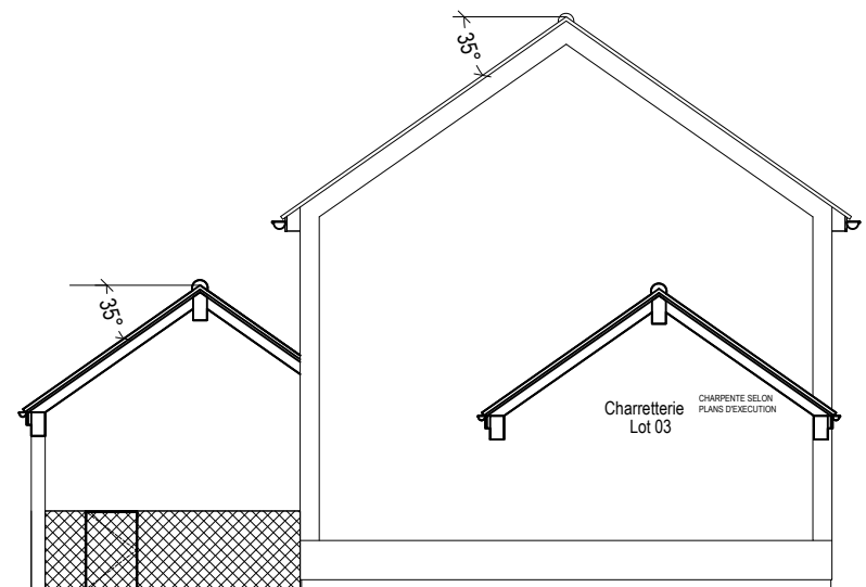
PIGNON GAUCHE
