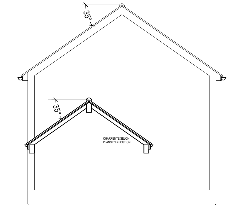
PIGNON DROIT
