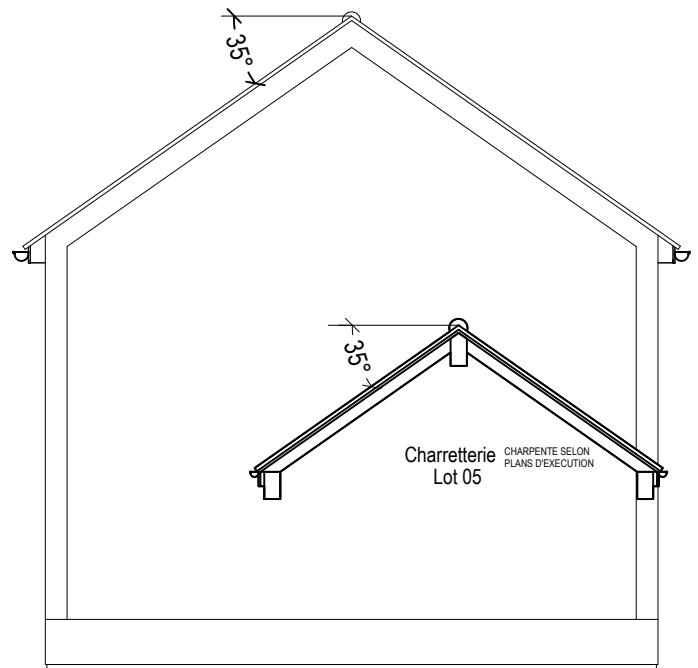
PIGNON GAUCHE
