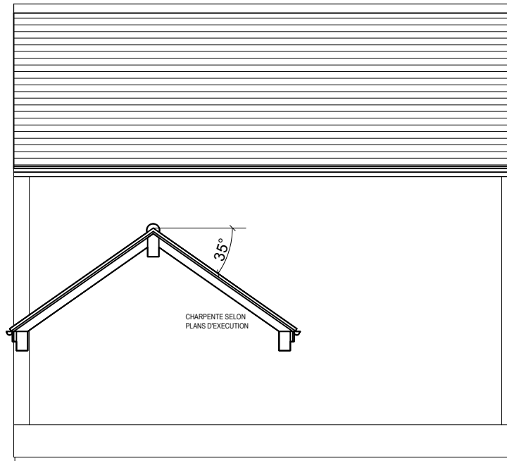
PIGNON DROIT
