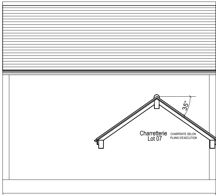
PIGNON GAUCHE
